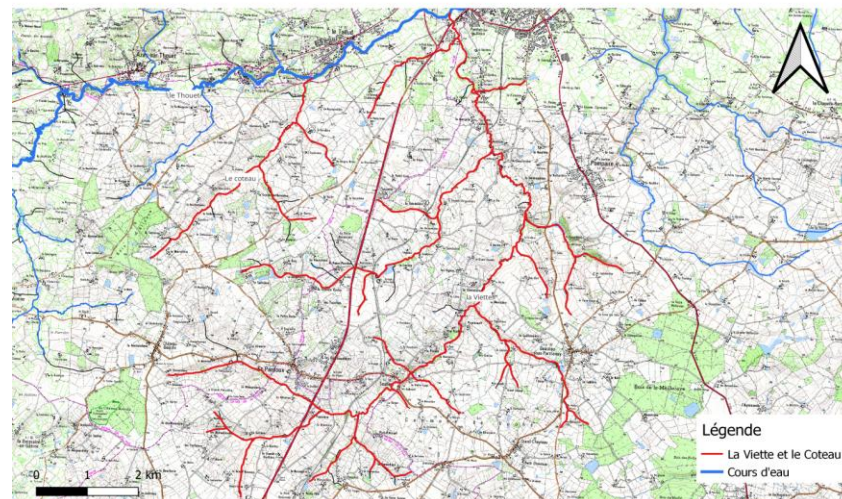
Réseau hydrographique de la Viette et du Coteau
